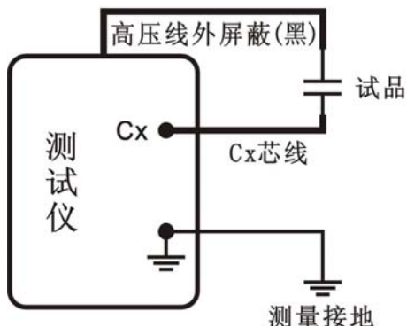
图 11 正接法
