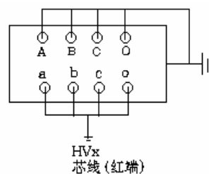
图 14 变压器接法
