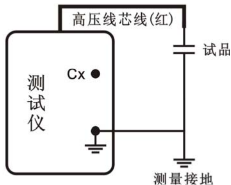
图 12 反接法
