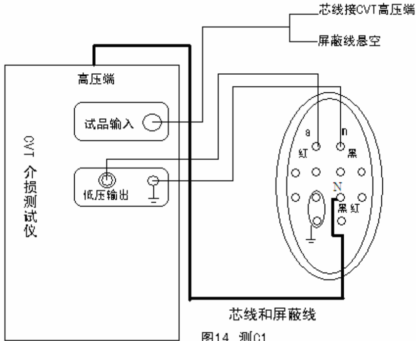
图14 测C1
