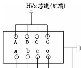
图 13 变压器接法
