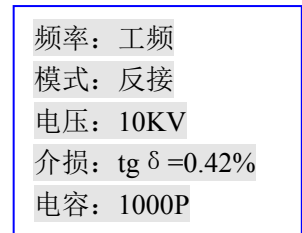
图10 打印结果
