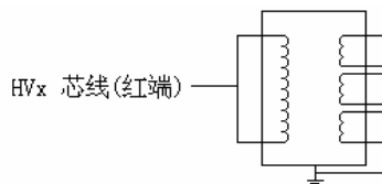
图7 PT接法
