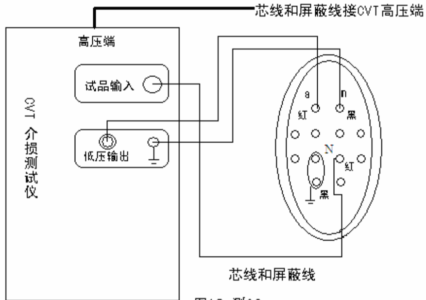
图13 测C2
