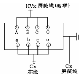
图 12 变压器接法
