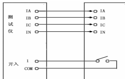
三相反时限接线
