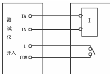
单相反时限接线
