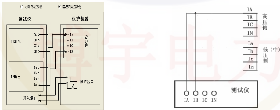
六相电流接线
